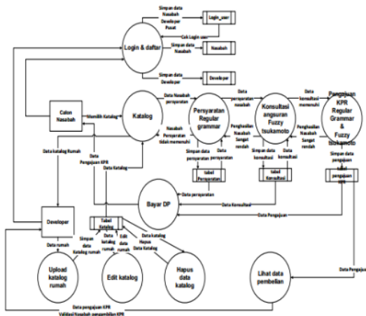
Gambar 1. DFD Analisis keputusan KPR
