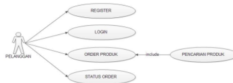
Gambar 1. Use Case Pelanggan
