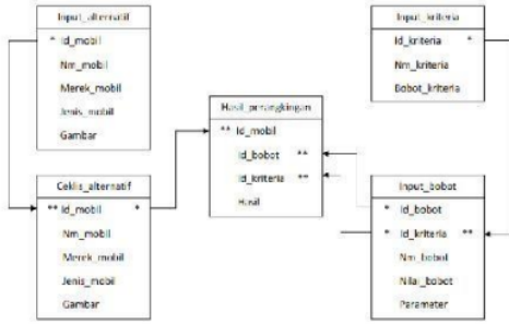
Gambar 3. Relasi Tabel
