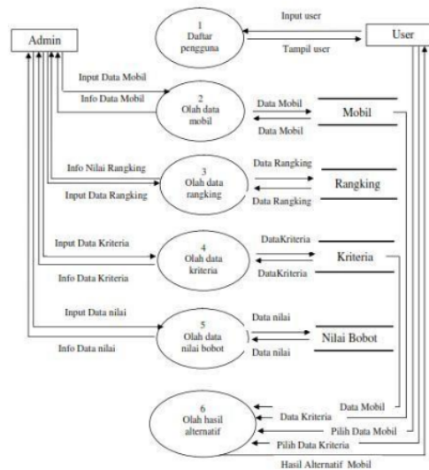
Gambar 2. DFD Level 1
