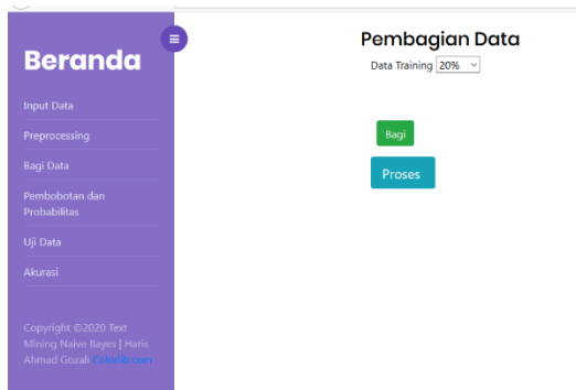
Gambar 4. Pembagian data training dan testing
